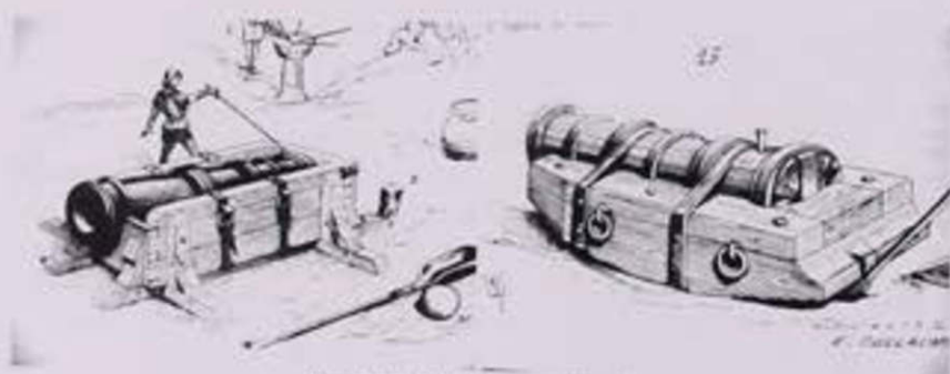
Bombardes placées sur un affût-chaîne. Dessins de Guillaumot publiés dans le Dictionnaire raisonné de l'architecture de Viollet-le-Duc.
